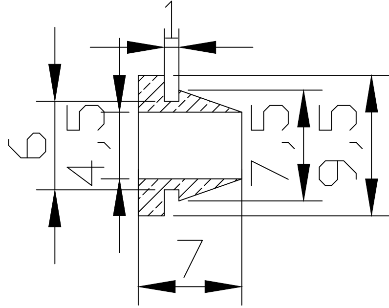
Sezione A-A
